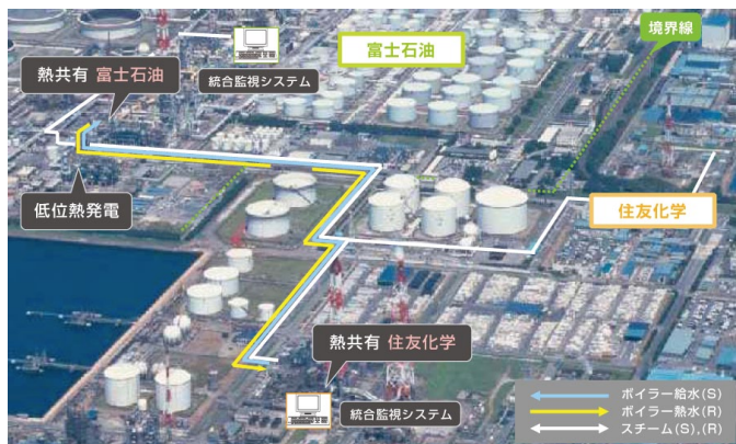
図6 富士石油と住友化学との共同事業。配管は片道約1.5km
