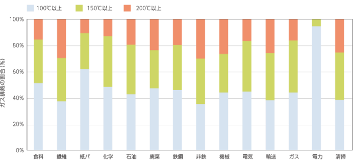
図A 業種別のガス排熱の割合。
